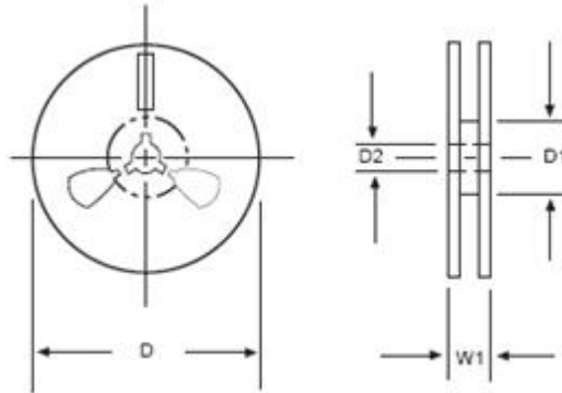
Fig 4. Reel dimensions
